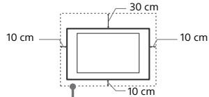
Television ympärille jätettävä minimi tila.
